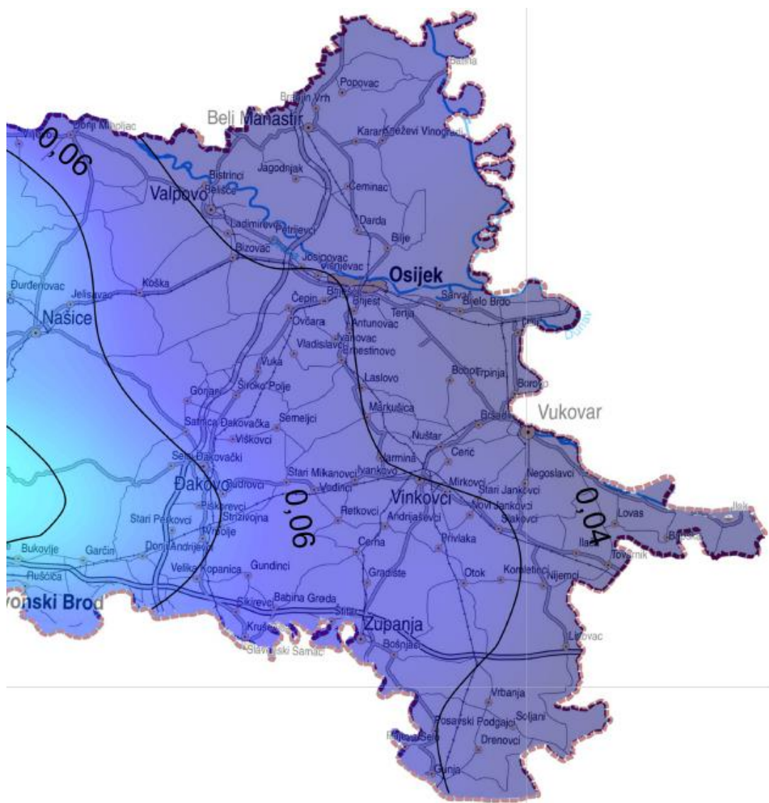
Slika 1-2 Seizmološka karta horizontalnih akceleracija u povratnom razdoblju 95 godina
